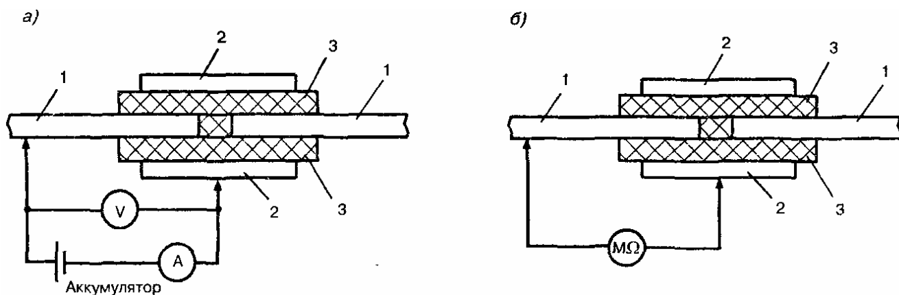
Рисунок 5 — Схема измерения сопротивления изоляции стыка ходового рельса
