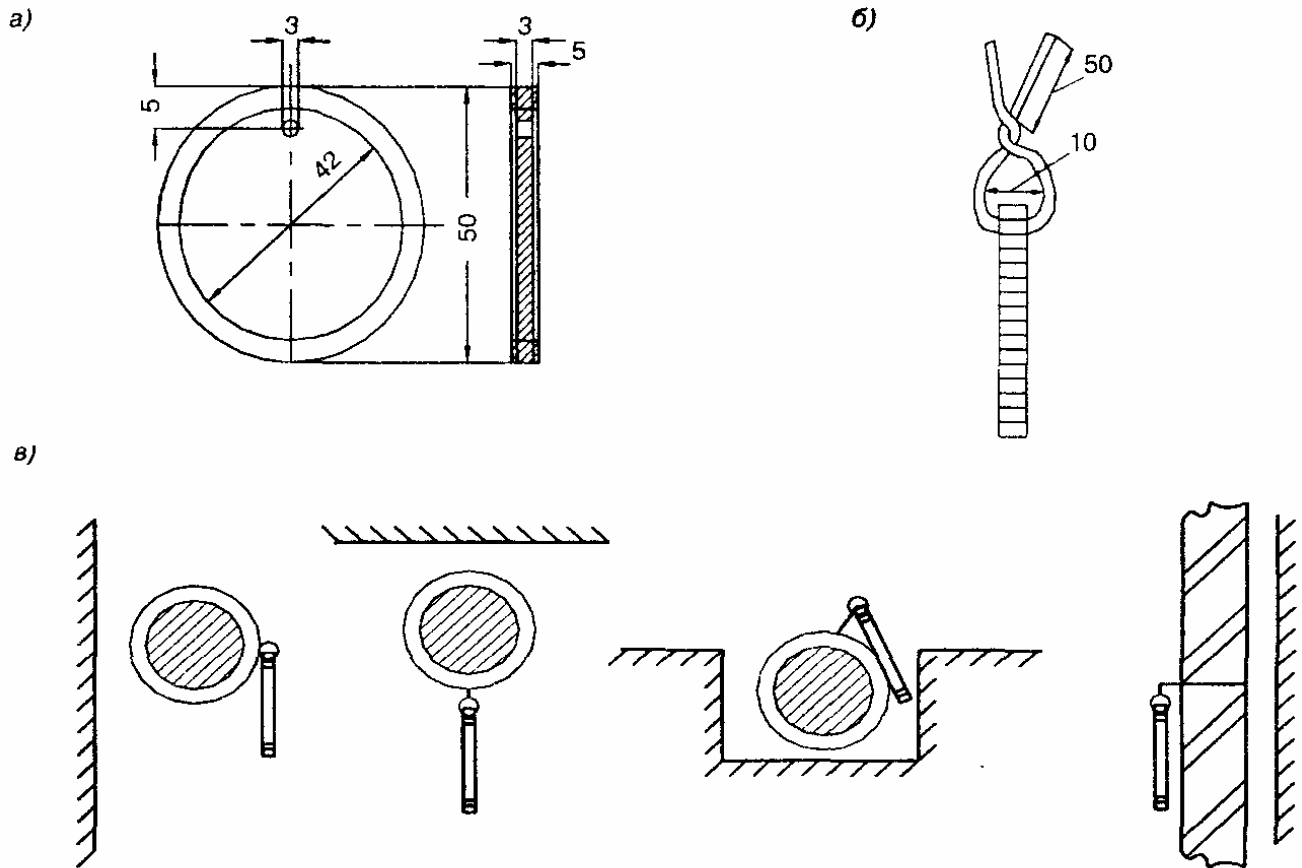
а — общий вид; б — узел подвешивания к проволоке; в — варианты подвешивания к кабелю
