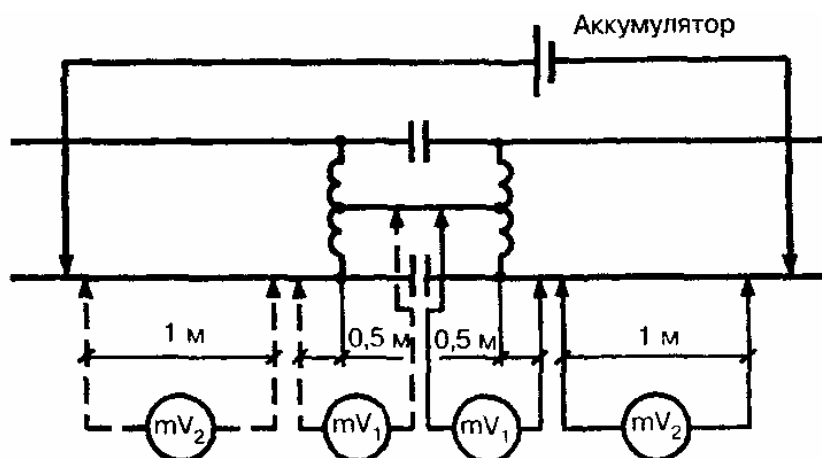
Рисунок 4 — Схема измерения сопротивления изолирующего стыка ходового рельса с ДТ "Рис. 4. Схема измерения сопротивления изолирующего стыка ходового рельса с ДТ"
