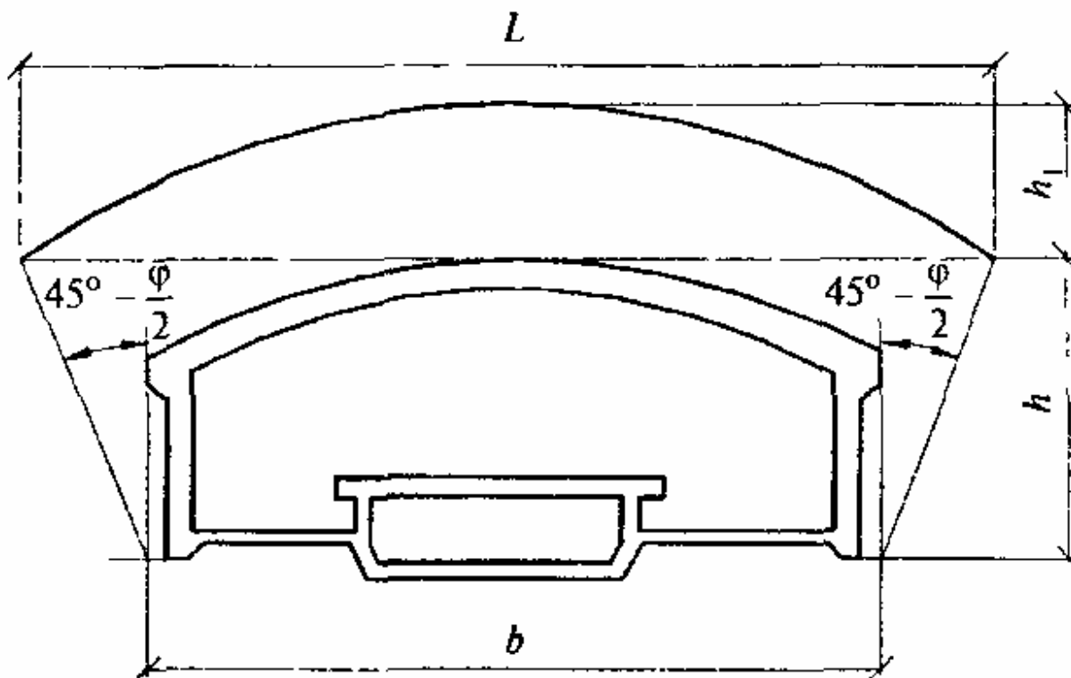
Рисунок 1 — Схема для расчета высоты свода обрушения
