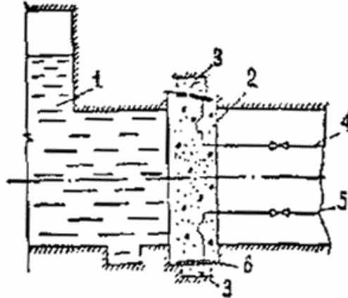
Рисунок 8 - Бетонная перемиčka с контурным гидрозатвором
