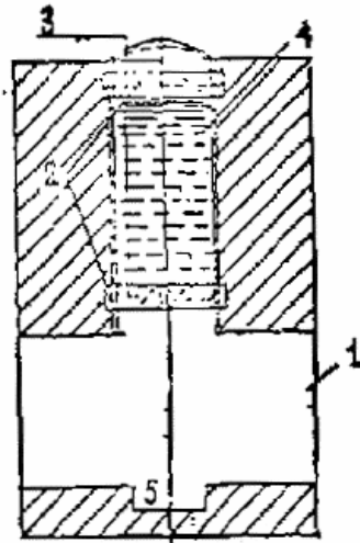
Рисунок 10 - Двойная бетонная перемычка с гидрозатвором, расположенная во вскрывающей выработке
