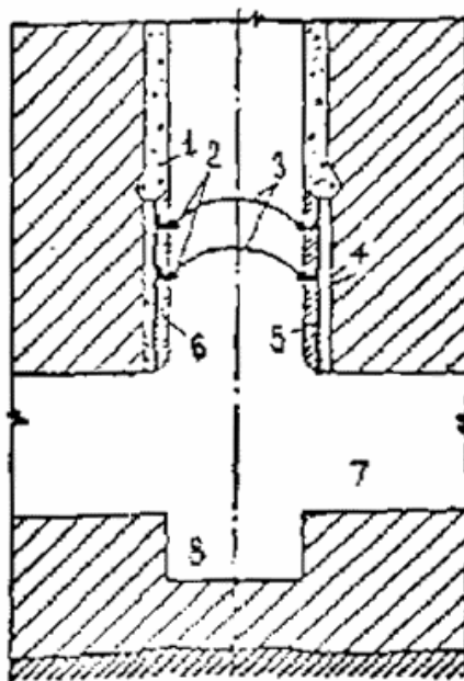
Рисунок 12 - Двойная металлическая перемычка, расположенная во вскрывающей выработке
