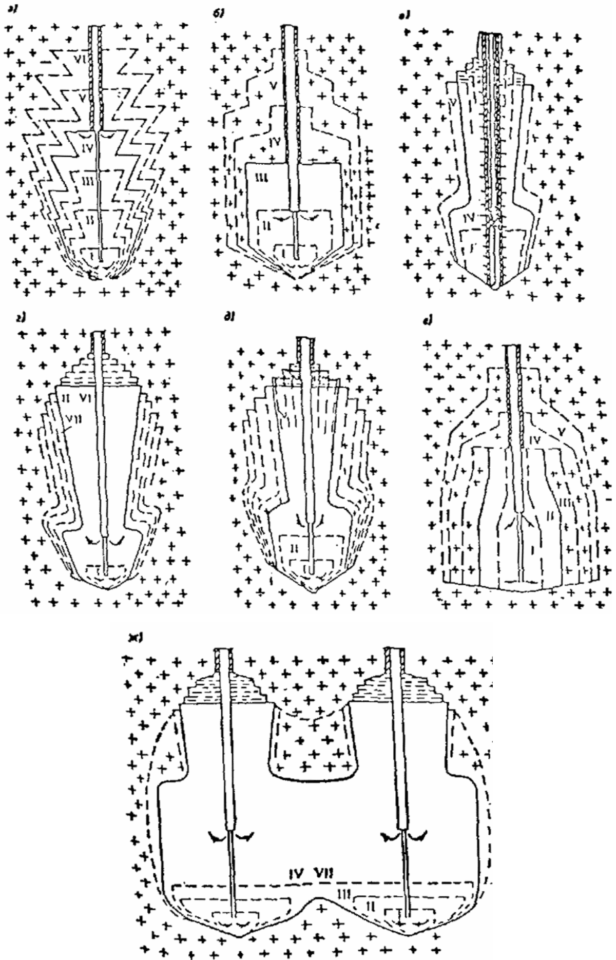
Рисунок 7 - Технологические схемы сооружения выработок-емкостей бесшахтных
