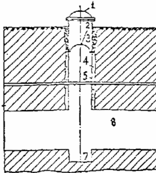
Рисунок 11 - Двойная металлическая перемычка, расположенная в верхней части ствола
