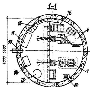
Черт. 127. Дренажная насосная станция
