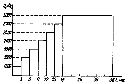
Черт. 149. Ступенчатый график откачки подземных вод к примеру 47
