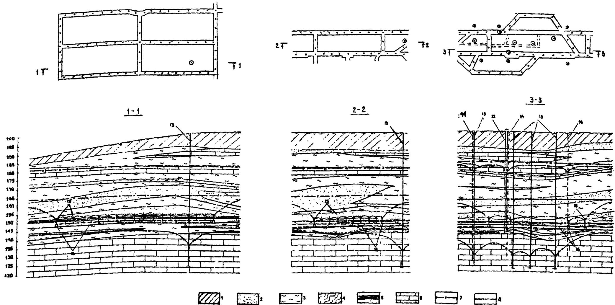
Черт. 31. Водопонижительная система шахтного поля
