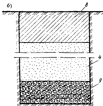
Черт. 120. Закрытые безтрубчатые дренажи
