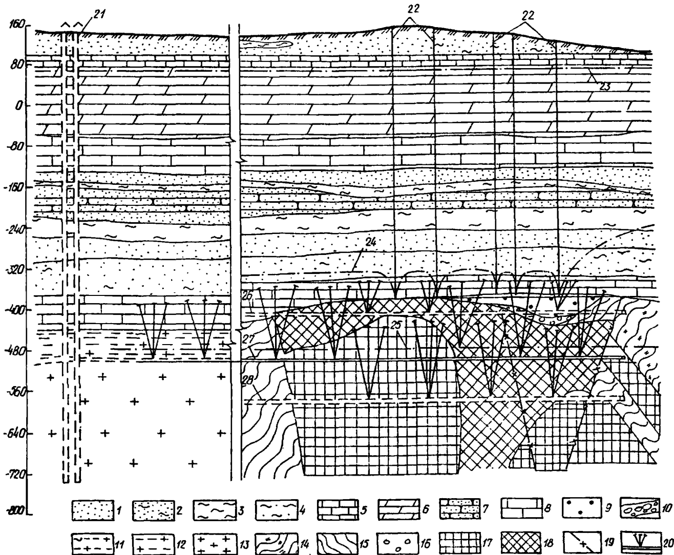
Черт. 30. Система водооплинения первоочередного участка. Разрез 1-1 (см. черт. 29)
