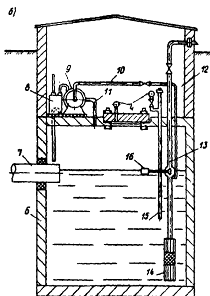
Черт. 128. Конструктивные схемы смотрового колодца с вакуумной камерой и насосной станцией с погружным центробежным насосом
