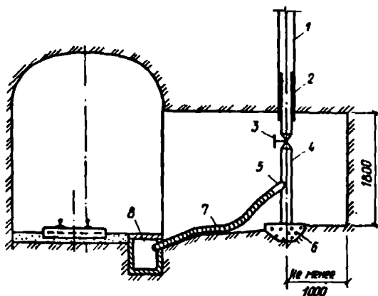
Черт. 51. Ходок к сквозному фильтру
