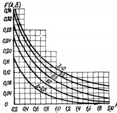
Рис.31. График функции F(\lambda; \bar{\Delta}_0) .
