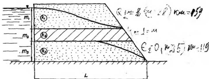
Рис.15. Схема к расчету фильтрации в случае трехслойного сложения откоса.
