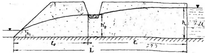
Рис.67. Схема к расчету несовершенной траншеи вблизи карьера.
