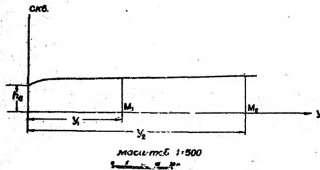
Рис.85. Депрессионная кривая по линии скважин.
