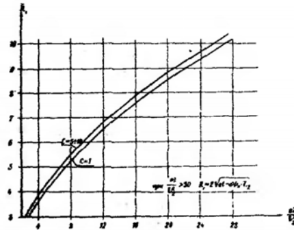
Рис.37. График для определения величины K_1 .
