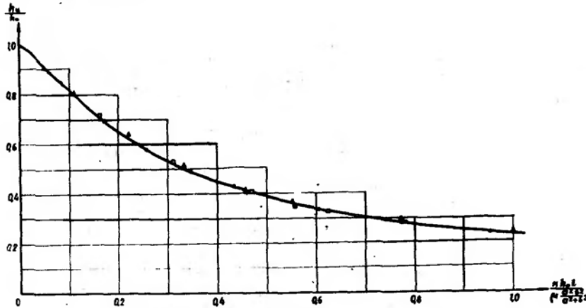
Рис.43. График функции h_u(t) .
