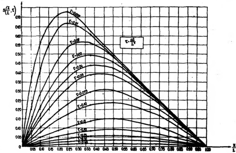
Рис.19б. График функции S(\frac{x}{L}; \tau) .
