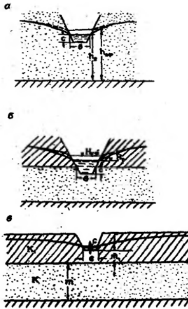
Рис.11. Схемы к расчету несовершенной траншеи.
