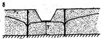
Рис. 26. Схемы к расчету линейных систем скважин вблизи совершенных котлованов.
