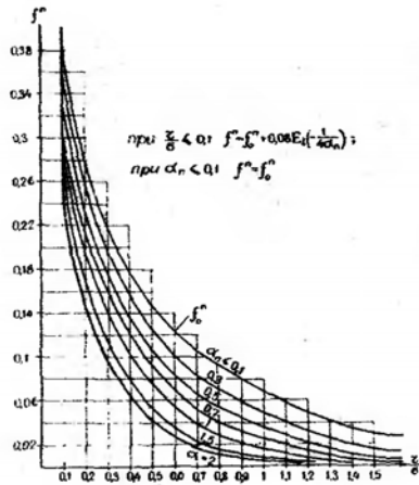
Рис.38. График функции f^n(\frac{r}{b}, \alpha_n) .
