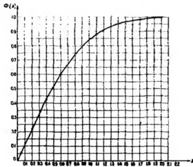
Рис.19а. График функции \Phi(\lambda) .
