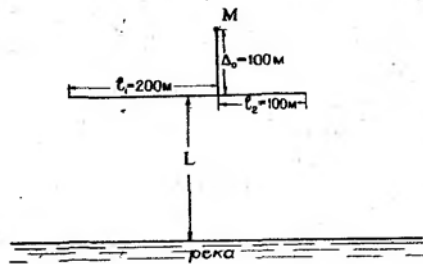
Рис.86. Схема к расчету линейного ряда водоопытных скважин у реки.
