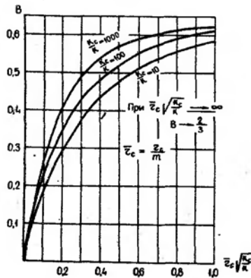
Рис.13 График для определения величины В в зависимости от параметра \frac{z_c \sqrt{K_c}}{k} .
