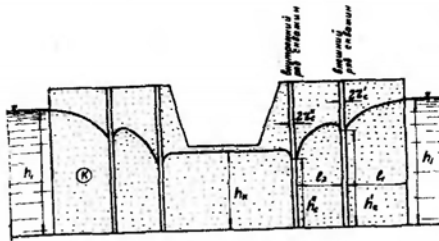
Рис. 27. Схема к расчету двухрядной установки скважин, расположенных по обеим сторонам несовершенного котлована.
