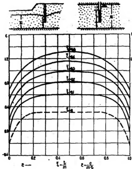
Рис.8. График к определению приведенного радиуса скважины.
