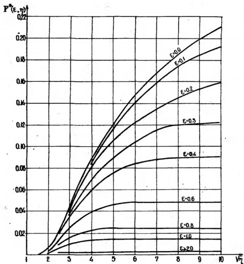
Рис.30. График функции F^*(\epsilon, \eta) .
