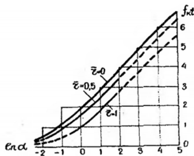
Рис.32. График функции f_{kt} .
