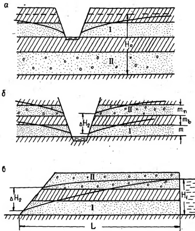
Рис.14. Схемы к расчету "перетекания".
