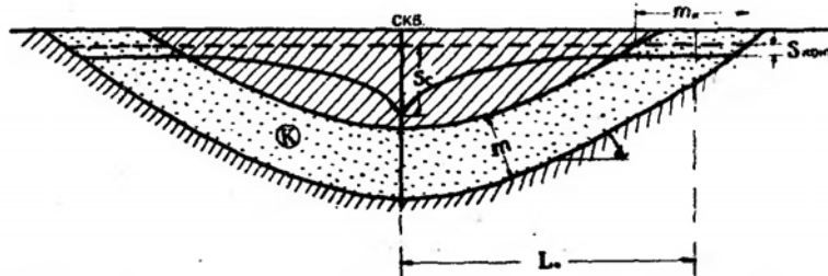
Рис.39. Ряд скважин в условиях мутьдообразного пласта.
