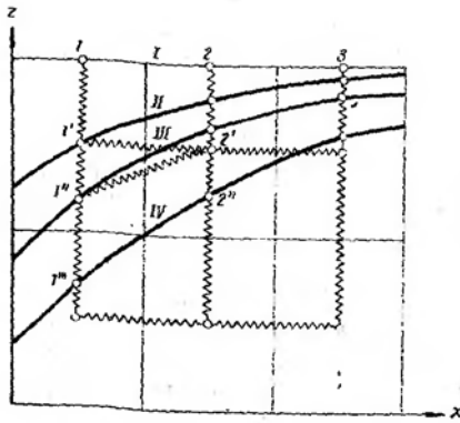
Рис.69. Схема к моделированию горизонтальных скважин.
