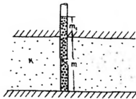
Схема скважины с песчано-гравийным заполнением
