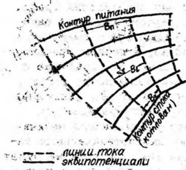
Рис.2. Схема ленты тока.
