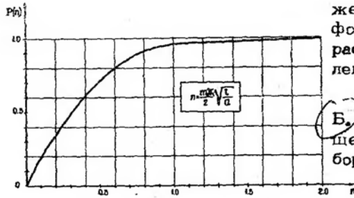
Рис.21. График функции P(n) .
