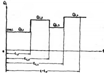
Рис.33. График изменения дебита i -ой скважины.
