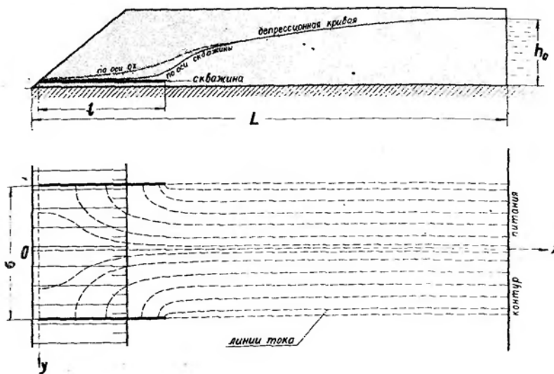
Рис.45. Схема к расчету горизонтальных дренажных скважин.
