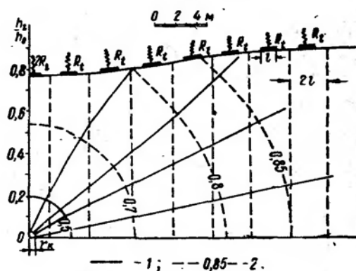
1-Линии тока, 2-эквипотенциали
