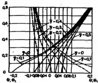
Рис.24. Графики функций \theta (пунктир) и \phi , (сплошные линии).
