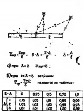
Рис.25. Схема к определению расчетного расстояния r_{эф} .
