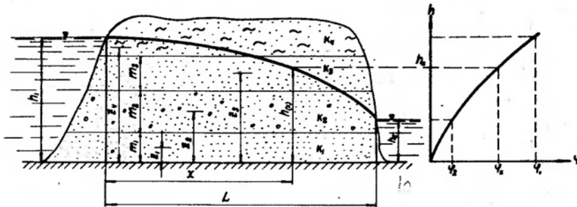
Рис.5. Схема к расчету безнапорной фильтрации в условиях многослойной толщи.
