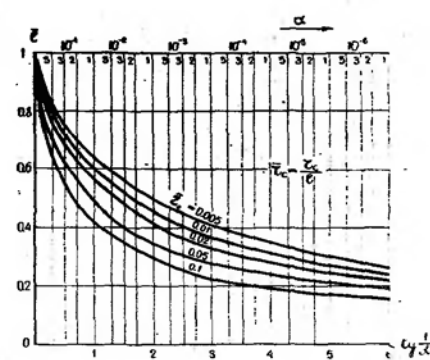
Рис.9. График для определения приведенного радиуса несовершенной скважины.
