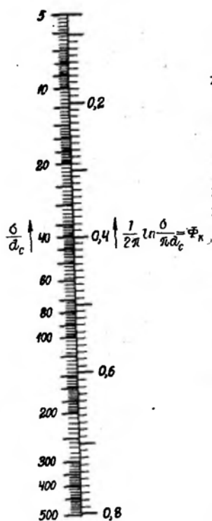
Рис.7. Номограмма для определения внутреннего сопротивления контура.
