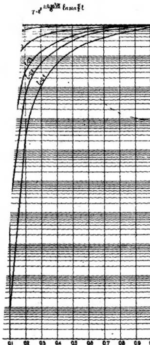
Рис. 10. График для определения коэффициента несовершенства дренажного контура.
