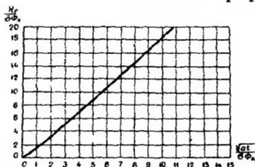
Рис.35. График для определения функции R_p
