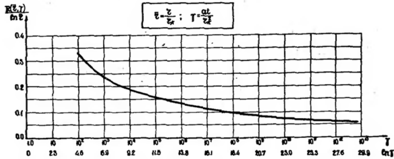
Рис.16. График функции R(r, \tau) .
