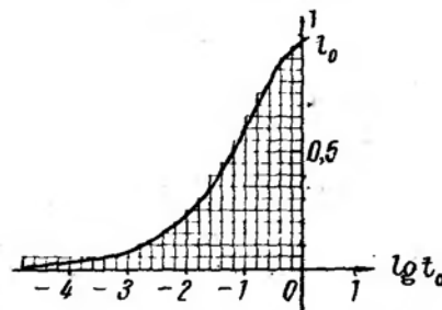
Рис.22. График l_0 = f(t_0) .
