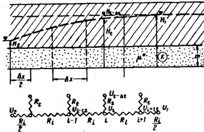
Рис.50. Схема к моделированию напорной неустановившейся фильтрации.
