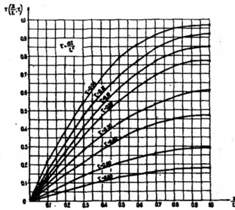
Рис.19в. График функции T(\frac{x}{L}; \tau) . применима при \frac{R_*}{r_k} > 5 .
