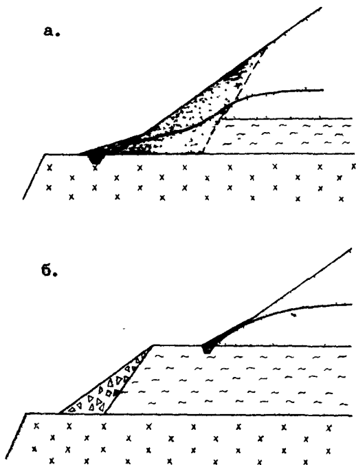
Рис. 13. Схемы пригрузки нерабочего уступа глинистых пород.
