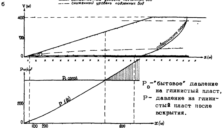
Рис. 4. Эпюры распределения давлений на глинистый пласт:
