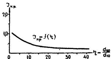
Рис. 5. График зависимости
