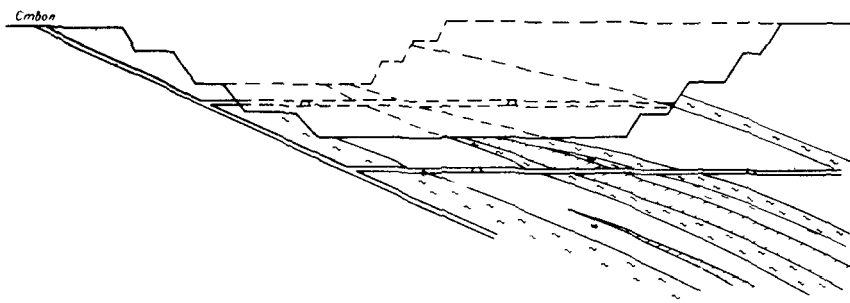
Рис. 20. Осушение карьера дренажными выработками, пройденными из наклонного ствола
