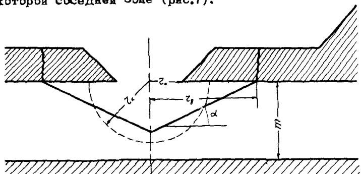
Рис. 7. Схема к расчету размеров деформированной зоны
