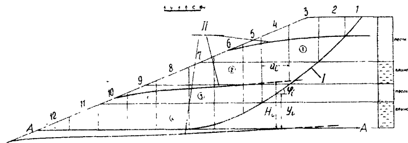
Рис.23. Схема к расчету устойчивости обводненного многослойного откоса
