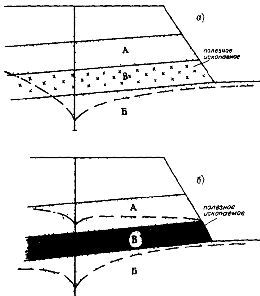
Рис. 19. Схемы дренажа рабочего борта водоупонизительными скважинами
