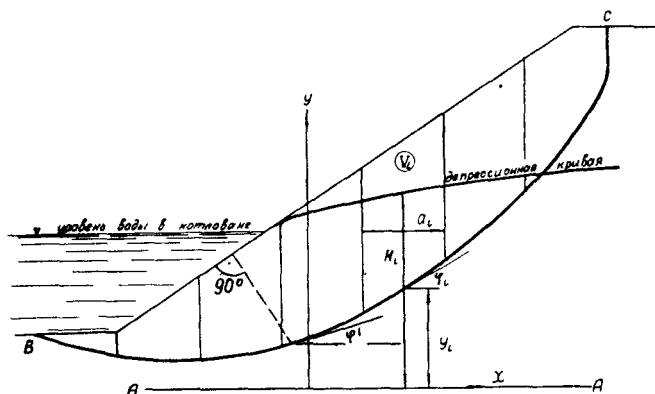
Рис. 2. Схема к расчету устойчивости обводненного откоса.
