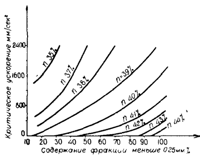
Рис. 8. Зависимость критического ускорения a_{кр} от механического состава и пористости песков ( n )
