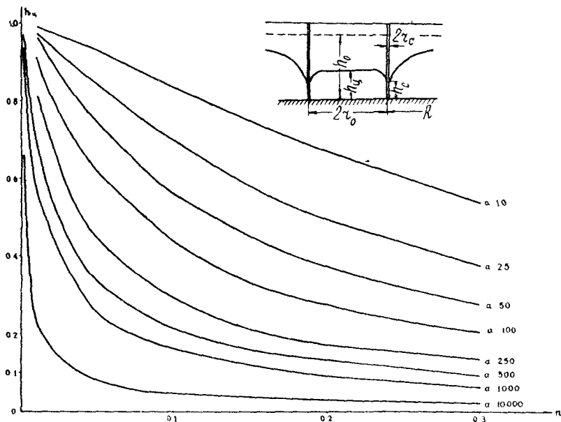
Рис. 15. График функции h_u = f(n) \left( h_u = \frac{h_d}{h_0} + \frac{\pi r_c}{r_0} a - \frac{r_0}{r_c} \ln \frac{R}{r_0} \right) при h_c^2 \ll h_0^2
