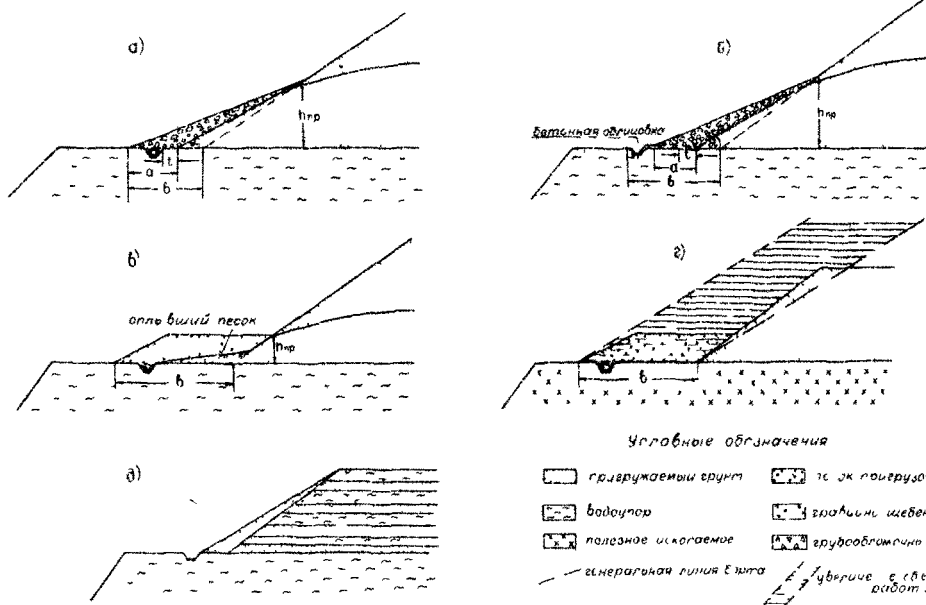
Рис. 12. Схемы дренажных пригрузок
