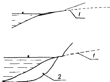
Рис. 10. Схема образования конусов выноса при различных углах наклона подводного откоса.
