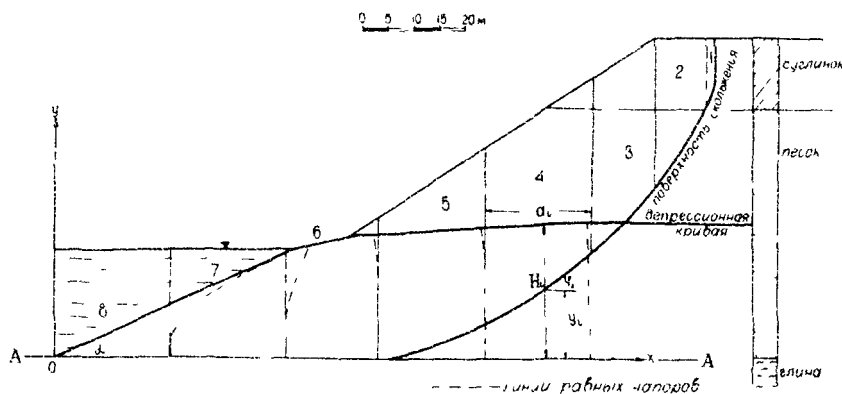
Рис.22. Схема к расчету устойчивости подтопленного откоса
