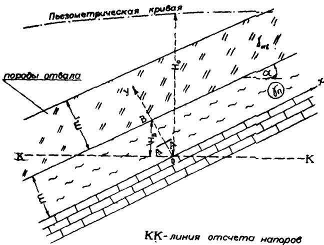
Рис. 1. Схема к определению "эффективных напряжений".
