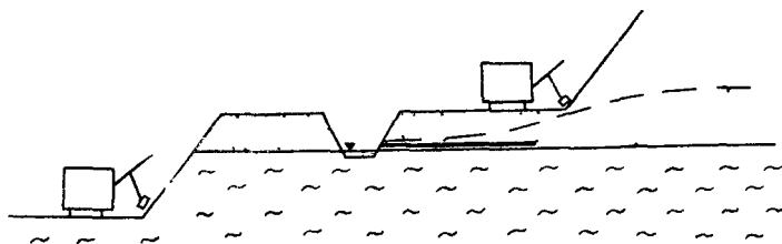
Рис. 17. Схема дренажа рабочего борта горизонтальными скважинами
