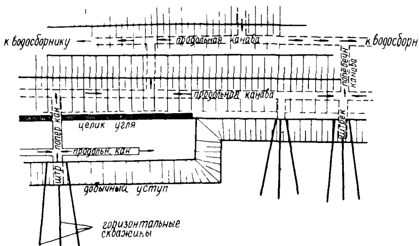
Рис. 21. Схема дренажа основания отвалов
