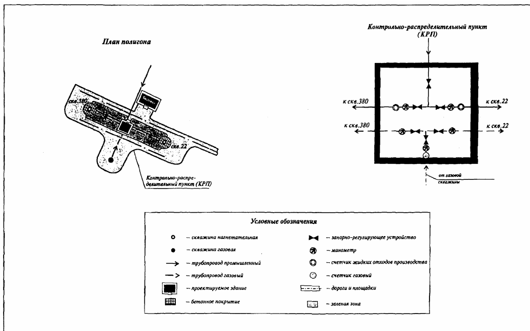
Рисунок 17.2 — Типовая схема обустройства полигона закачки жидких отходов производства
