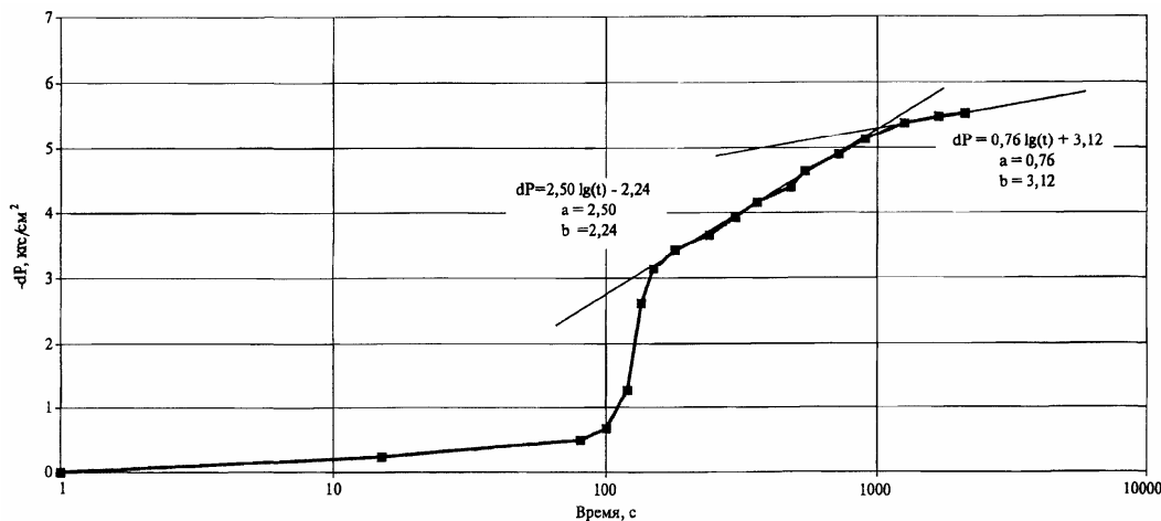
Рисунок 6.1 — Кривая восстановления забойного давления
