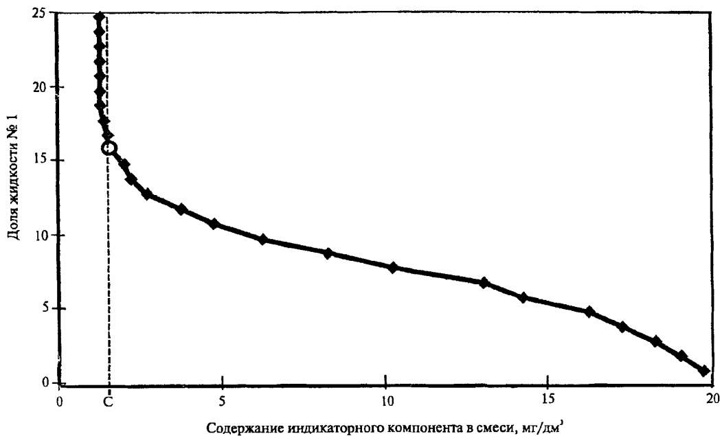
Рисунок 8.2 — График смешения жидкостей
