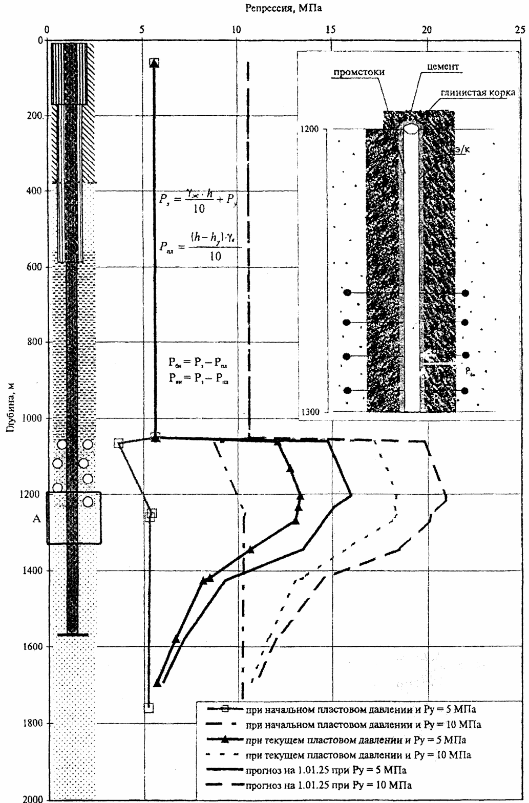
Рисунок 13.1 — Изменение боковой нагрузки на эксплуатационную колонну и цементный камень
