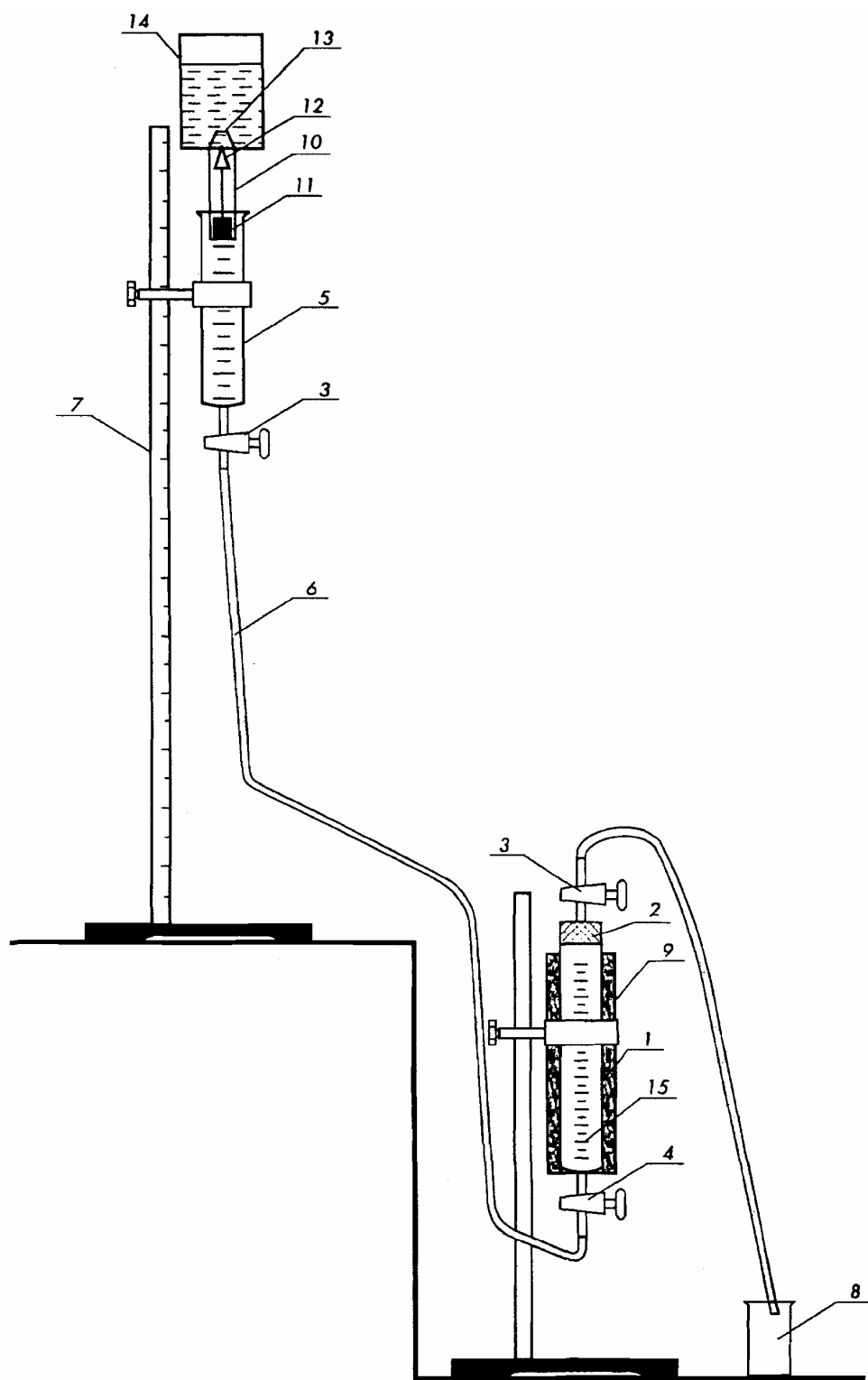
Рисунок 8.1 — Устройство для исследования совместимости систем "жидкость-жидкость" и "жидкость-порода"
