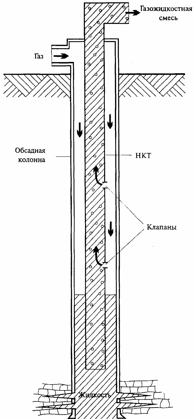
Рисунок 17.1 — Газлифт
