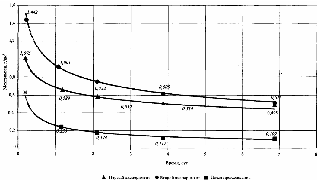
Рисунок 5.2 — Динамика выпадения в осадок механических примесей из жидких отходов производства
