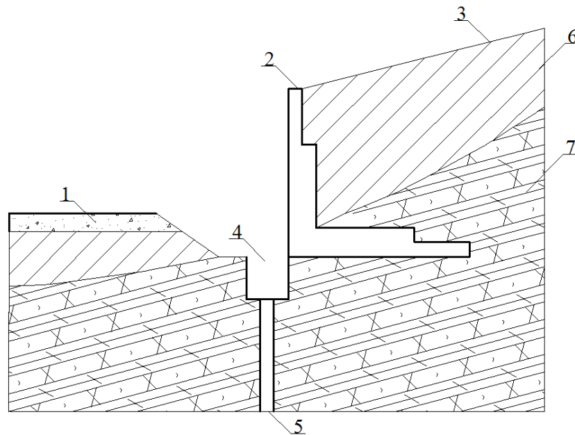
Рисунок 1 – Схема расположения шурфа и скважины около противооползневого сооружения: 1 – автомобильная дорога; 2 – подпорное сооружение уголкового типа; 3 – поверхность оползневого склона; 4 – шурф; 5 – скважина в шурфе; 6 – делювиальные суглинки; 7 – коренные породы флишевой формации
